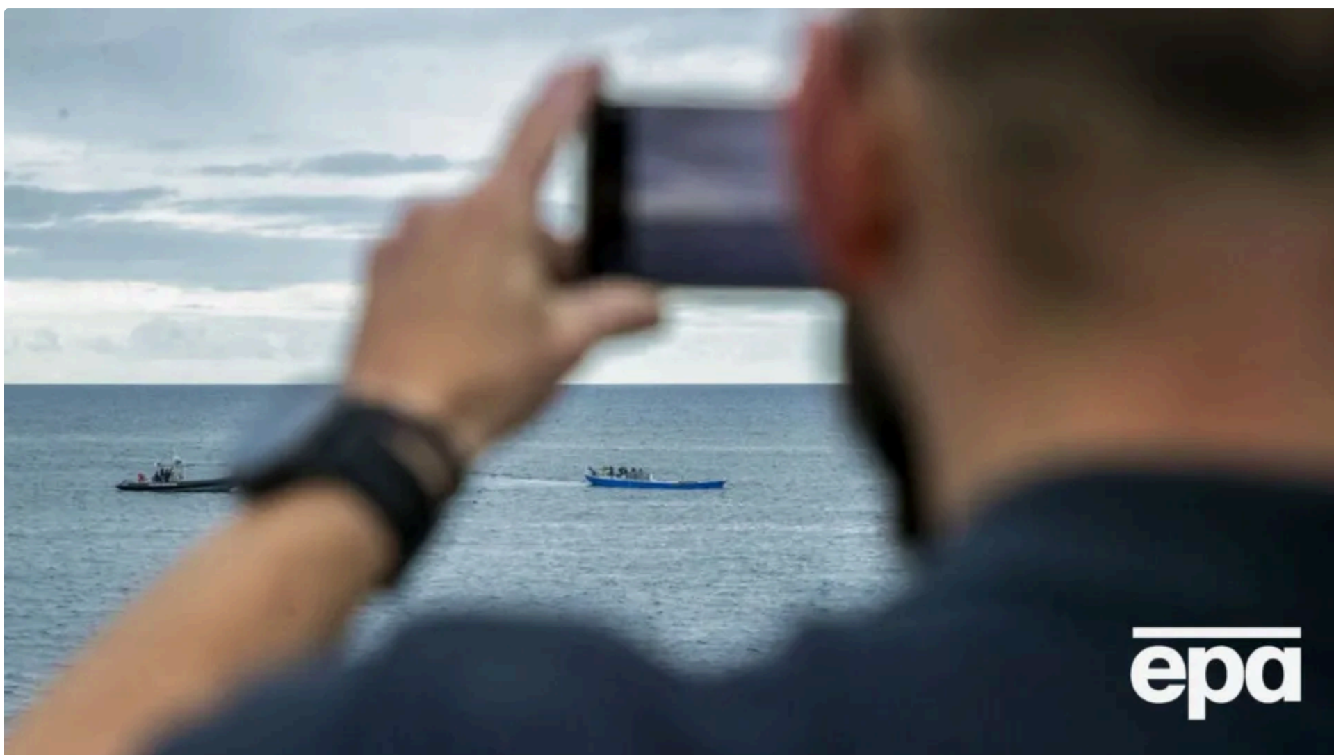
Професор Рамсторф вважає, що причиною утворення "холодної плями" стали зміни в роботі Атлантичної меридіональної перекидалної циркуляції Фото: ERA
