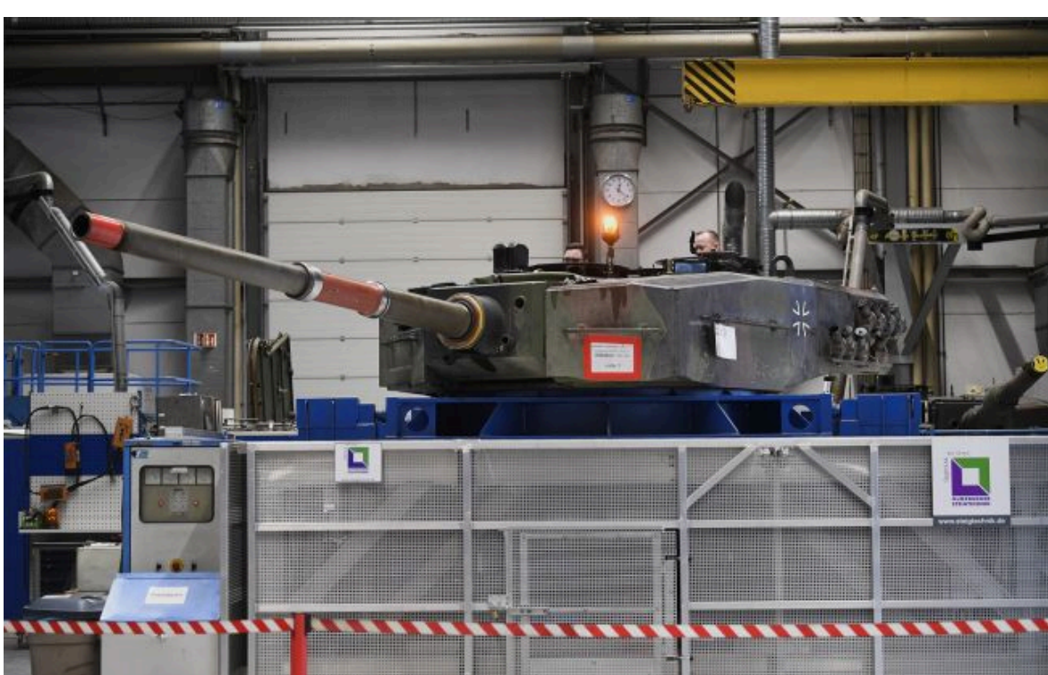
Фото: виробництво танка Leopard 2 на заводі Rheinmetall (Getty Images)
