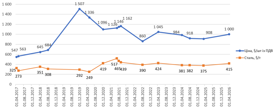
Ціна суцільнокатаних коліс Ø957 мм ст. 175 мм від "Інтерпайпу" для "ЦЗВ" у порівнянні зі світовою ціною сталі
